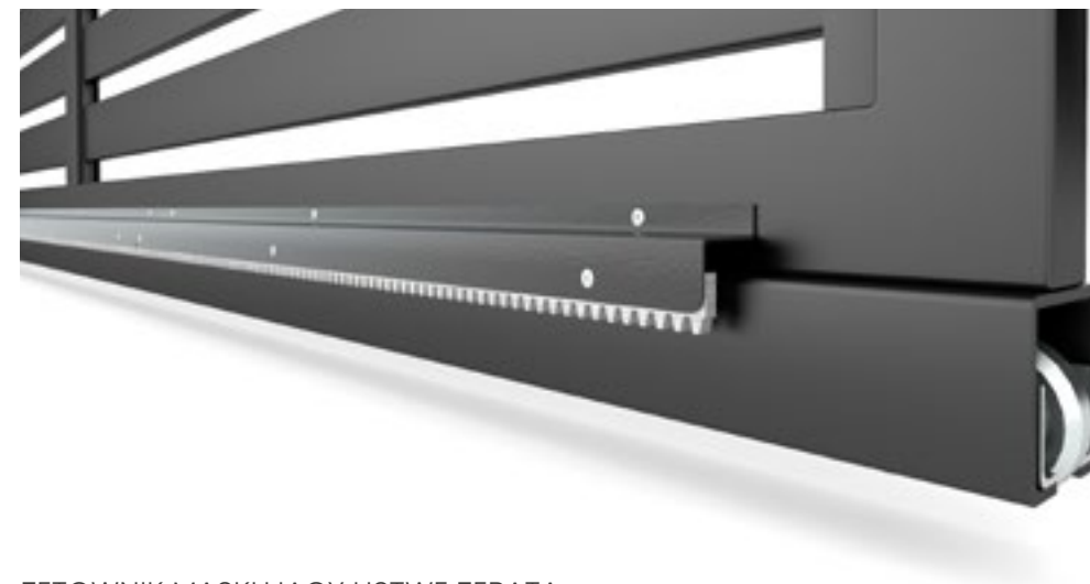
ZETOWNIK MASKUJĄCY LISTWĘ ZĘBATĄ
